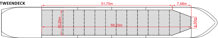
TWEEDECK
